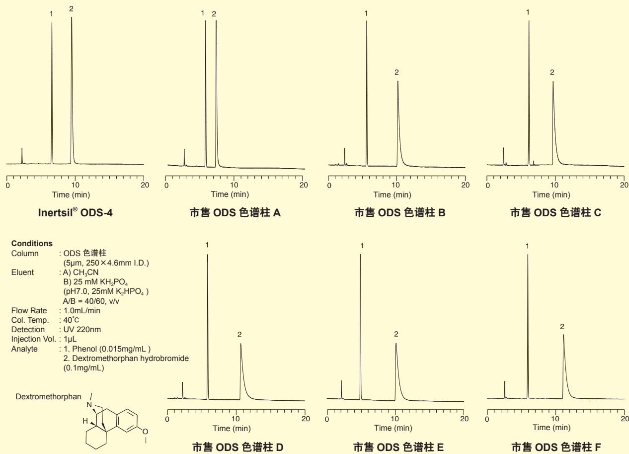
图 1: 与市售 ODS 色谱柱的强碱性化合物分析比较
